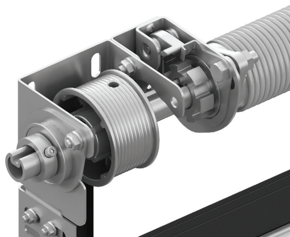
Detajl vzmeti.
